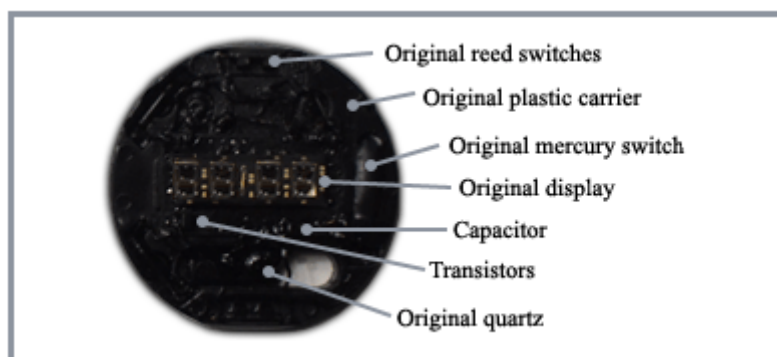
Abb. 1: Komponenten des SASM32 Moduls
